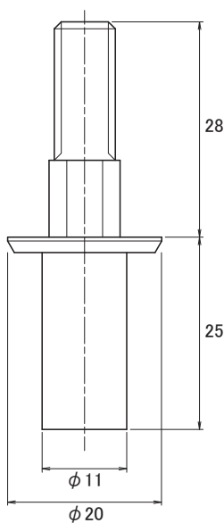
寸法図
