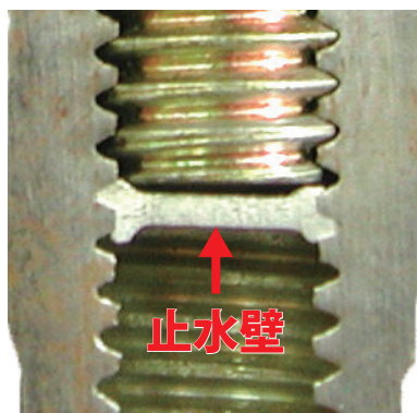
止水壁付タイプ断面
